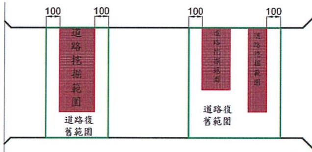
5.八公尺以上道路(沿行車方向開挖-雙車道)
