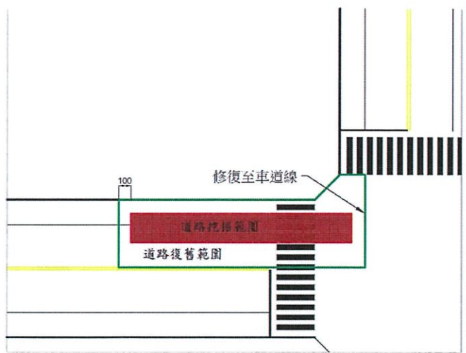
6.八公尺以上道路(到路口)
