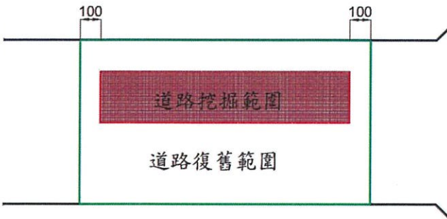
1.未達八公尺道路(沿行車方向開挖)
